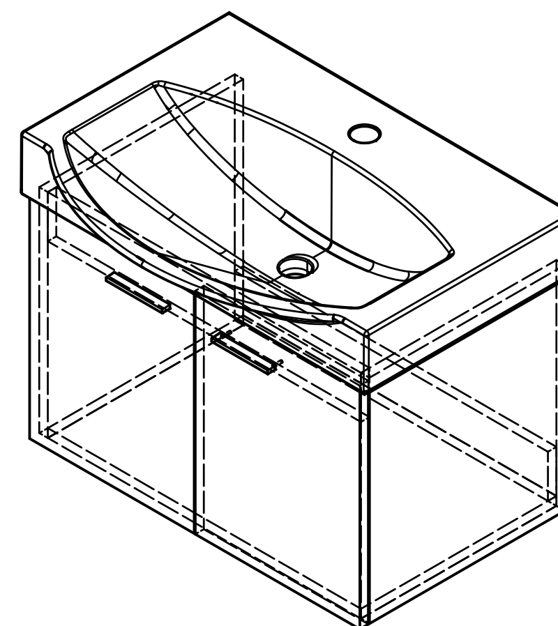
51067 - bílá 51068 - mali wenge 620x400x385 - skříň 650x495x490 - celek
